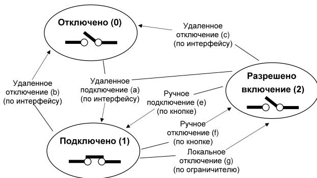
Рисунок 1.4 – Режим работы 2. Разрешены переходы a, b, c, e, f, g.
