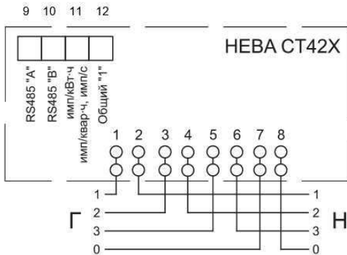
Схема подключения счетчика НЕВА СТ421 непосредственно к сети.
