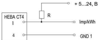
Рисунок 2.1 – Подключение испытательных выходов счетчиков HEBA CT4
