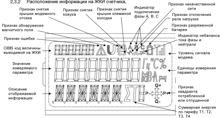
Рисунок 2.3 – Расположение информации на индикаторе
