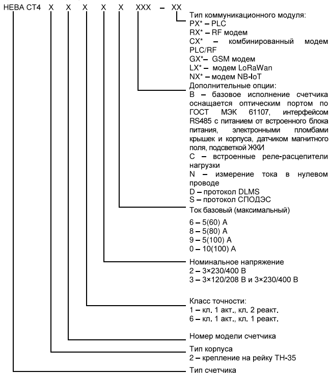
Рисунок 1.1 – Структура условного обозначения счетчиков НЕВА СТ421.
