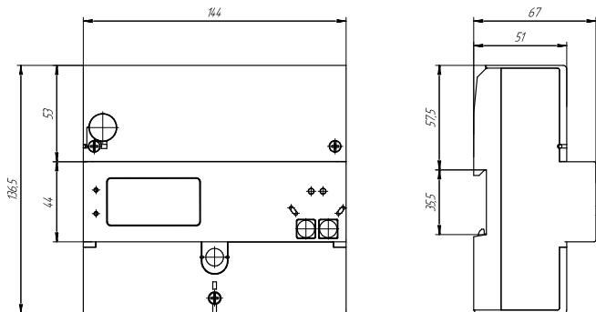
Внешний вид и габаритные размеры счетчика НЕВА СТ421
